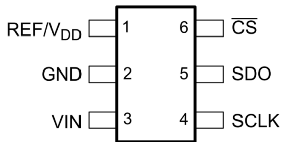
引脚图
