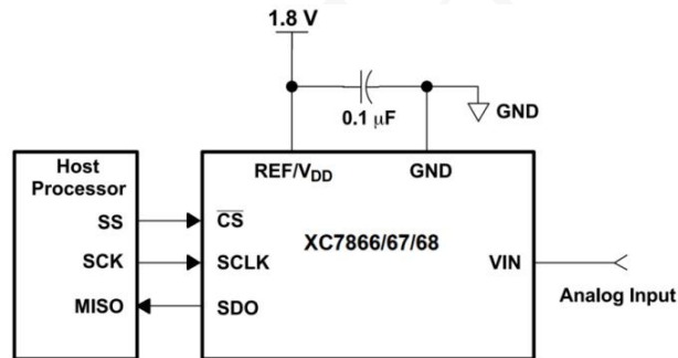
电路连接图
