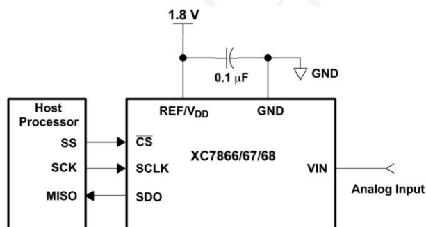
电路连接图
