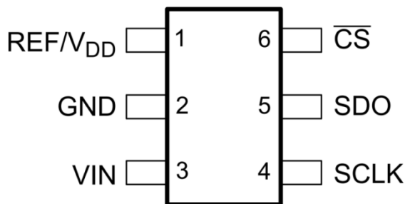
引脚图
