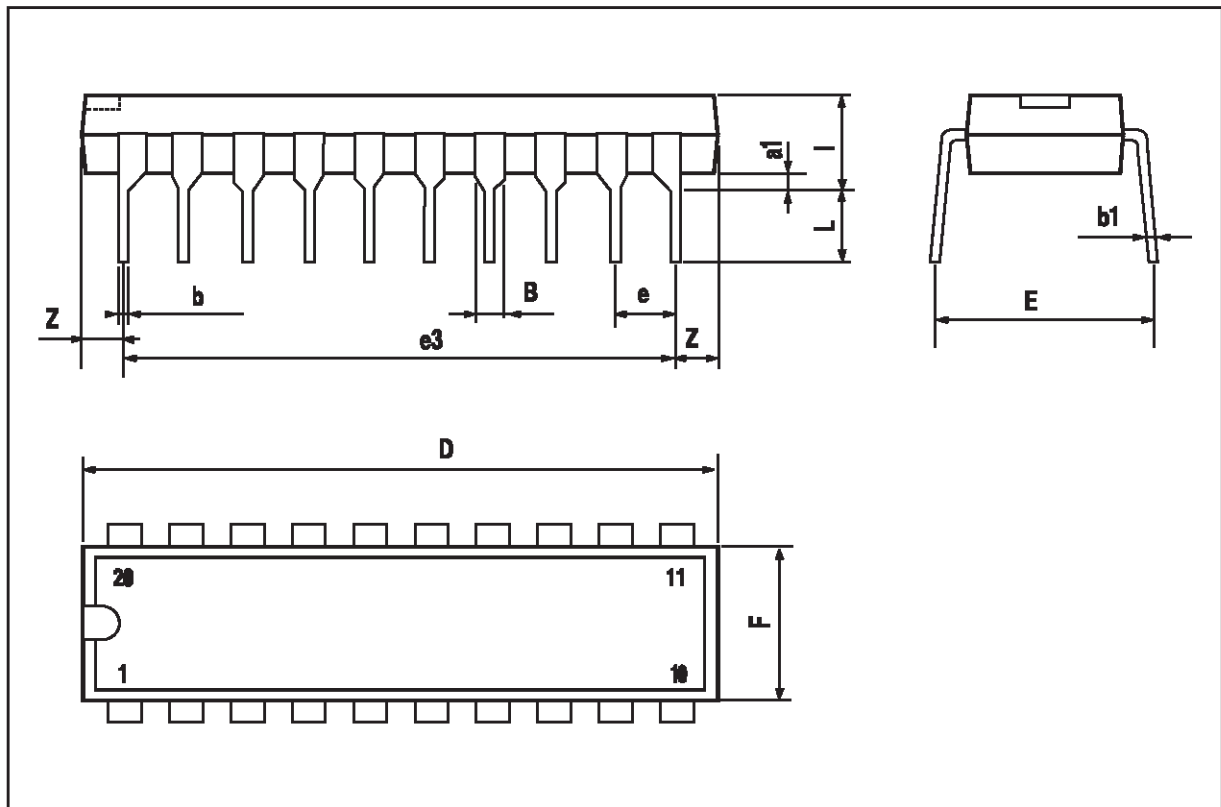
DIP20
