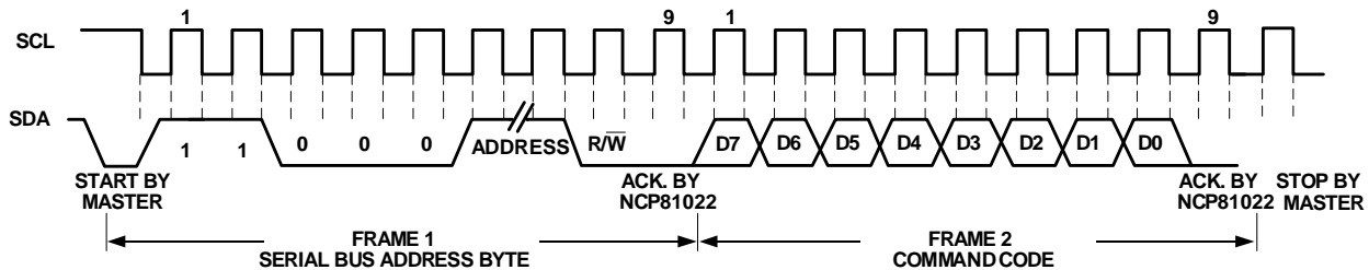
Figure 21. Send Byte
