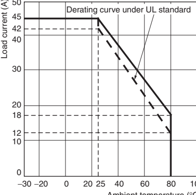
G3PB-445B-3-VD G3PB-445B-2-VD
