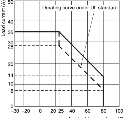
G3PB-435B-3-VD G3PB-435B-2-VD
