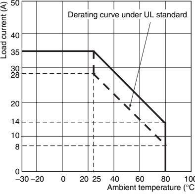
G3PB-235B-3-VD G3PB-235B-2-VD
