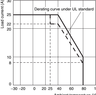
G3PB-425B-3-VD G3PB-425B-2-VD
