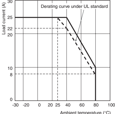
G3PB-225B-3-VD G3PB-225B-2-VD
