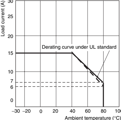
G3PB-415B-3-VD G3PB-415B-2-VD
