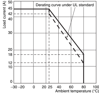
G3PB-245B-3-VD G3PB-245B-2-VD
