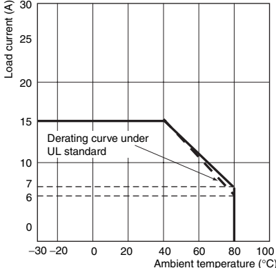
G3PB-215B-3-VD G3PB-215B-2-VD
