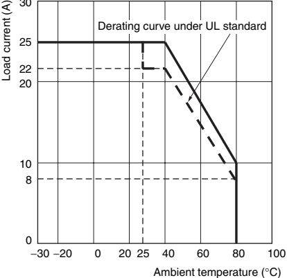
G3PB-425B-3-VD G3PB-425B-2-VD
