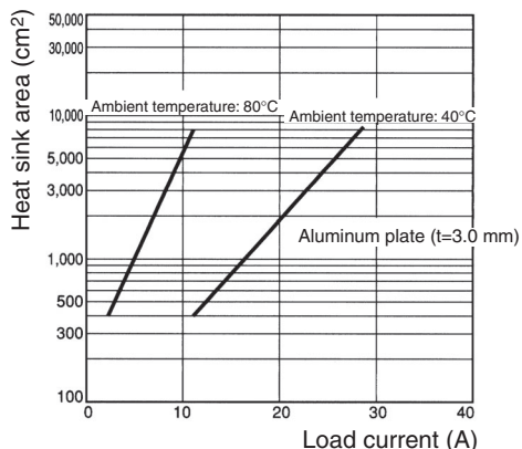
G3PB-225B-3H-VD
