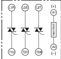
G3PB-245B-3-VD
