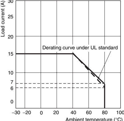
G3PB-415B-3-VD G3PB-415B-2-VD
