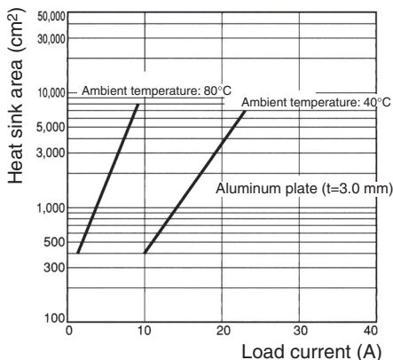
G3PB-425B-3H-VD
