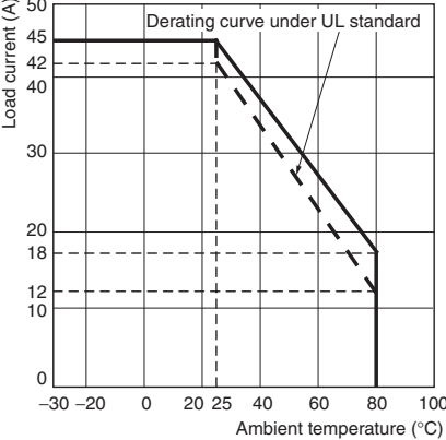
G3PB-445B-3-VD G3PB-445B-2-VD
