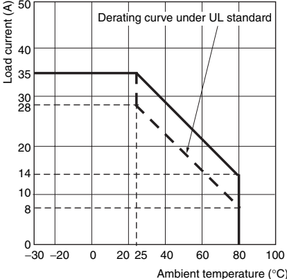
G3PB-435B-3-VD G3PB-435B-2-VD
