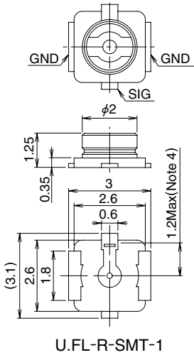
U.F.L-R-SMT-1
