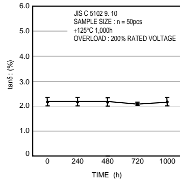
Fig.20 tan δ
