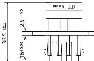
Receptacle, 12 poles
