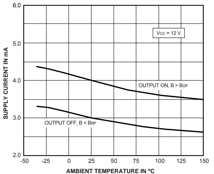
Dwg. GH-028-5
