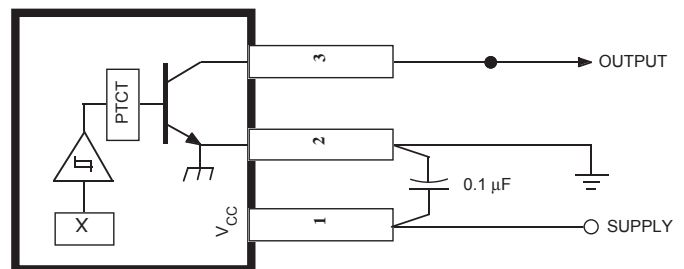
Dwg. EH-013
