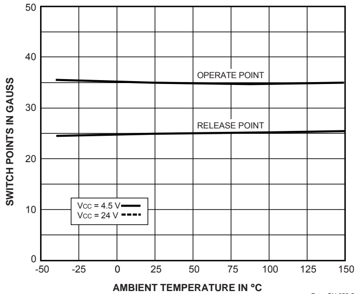
Dwg. GH-026-5
